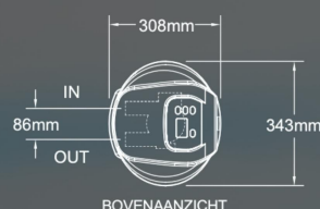
BOVENAANZICHT
