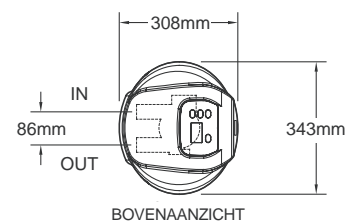
BOVENAANZICHT
